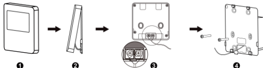
Abb. 4.9: Abbauen des Wandcontrollers
