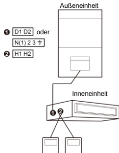
Abb. 4.5: Zwei Wandcontroller steuern eine Inneneinheit
